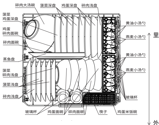
下层碗架摆放
